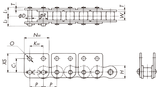
WSK2アタッチメント
