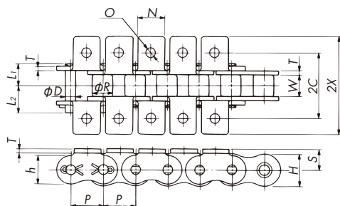
K1アタッチメント
