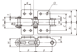
K2アタッチメント
