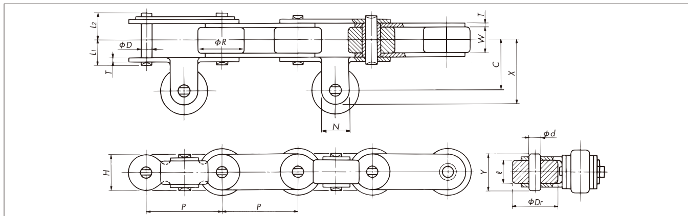
■アタッチメント寸法表
