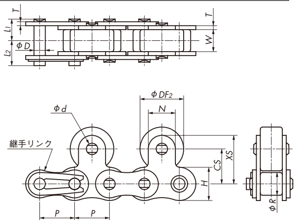
トップローラの取付間隔が2リンク毎以上の場合
