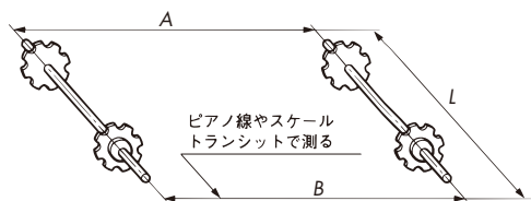
図2. 軸の平行度
