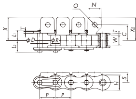
A1アタッチメント
