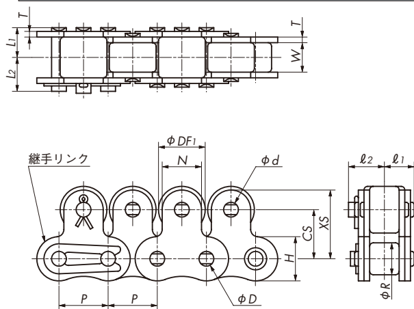
トップローラの取付間隔が1リンク毎の場合
