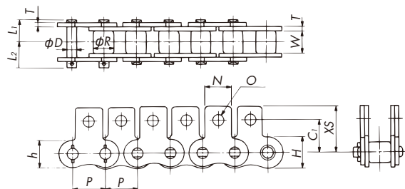
SK1アタッチメント
