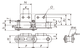
A2アタッチメント
