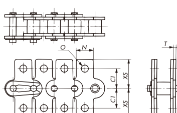
SKK1アタッチメント
