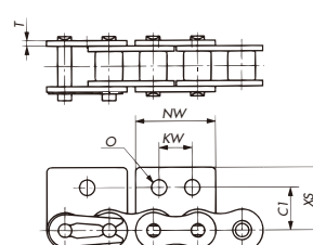
WSA1、WSA2アタッチメント
