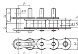
EPアタッチメント
