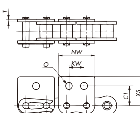
WSK1、WSK2アタッチメント
