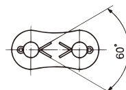
図22. 割ピンの開脚
