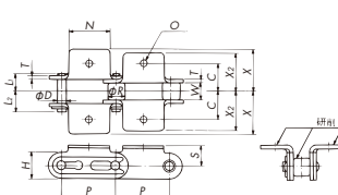
K1アタッチメント
