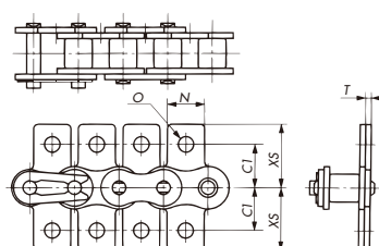
SAA1アタッチメント
