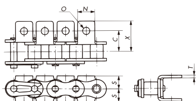
AA1アタッチメント
