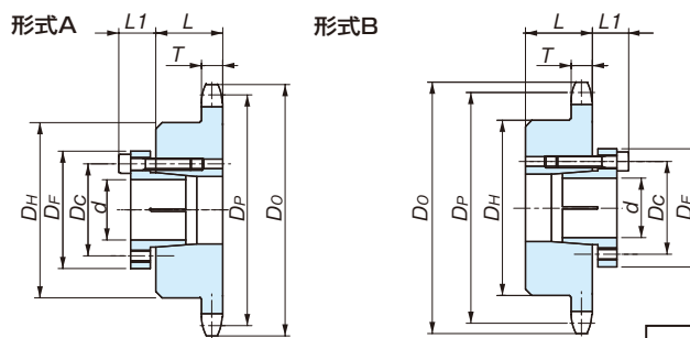
◆ S タイプ ロックスリーブ寸法
