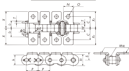
K1アタッチメント
