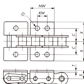
WK1、WK2アタッチメント
