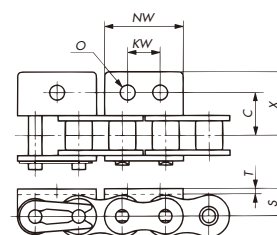
WA1、WA2アタッチメント
