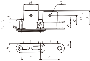
A1アタッチメント
