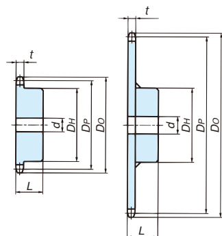
(削出し仕様) (溶接仕様) 1 B形
