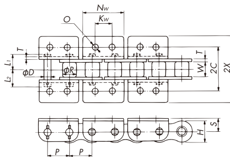
WK2アタッチメント
