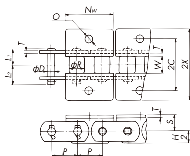
WK1アタッチメント
