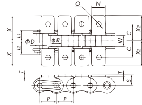
K1アタッチメント
