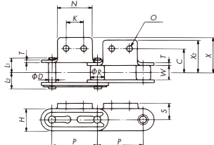
A2アタッチメント
