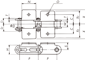
K1アタッチメント
