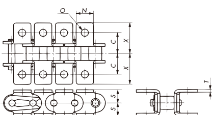
KK1アタッチメント
